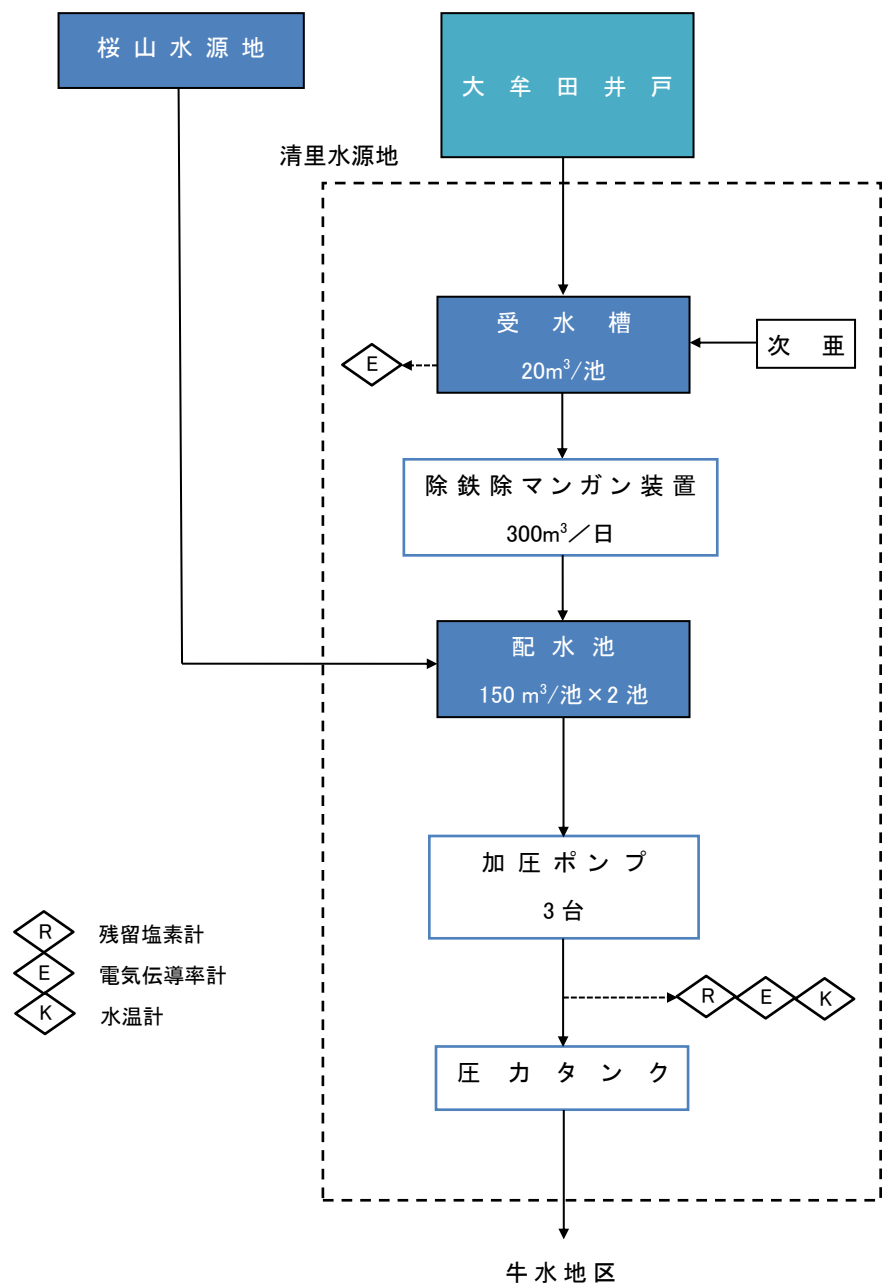
図 3.2-8 清里水源地浄水処理フロー
