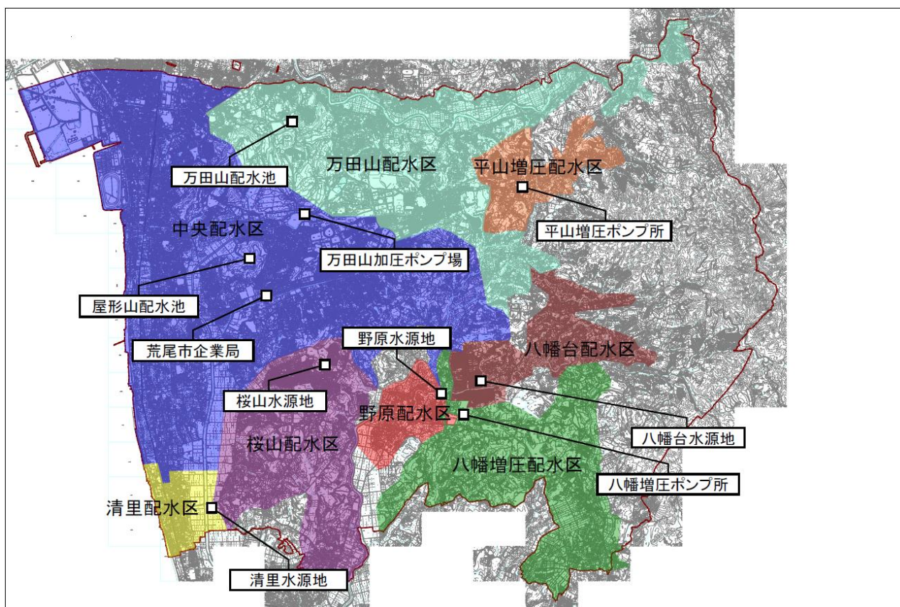
図 3.2-1 配水区分図
