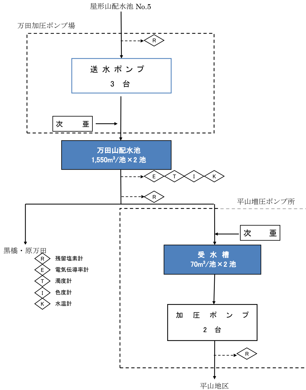
図 3.2-4 万田加圧ポンプ場～平山増圧ポンプ所浄水処理フロー
